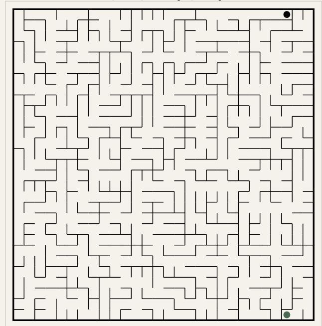
Puzzle 4 (28x29)
