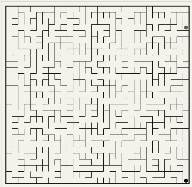
Puzzle 7 (30x29)
