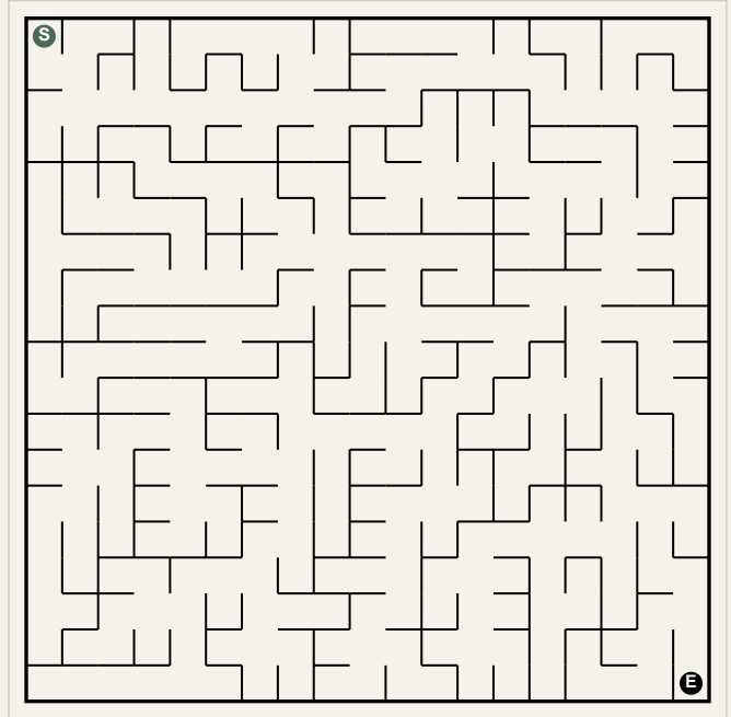
Puzzle 2 (19x19)
